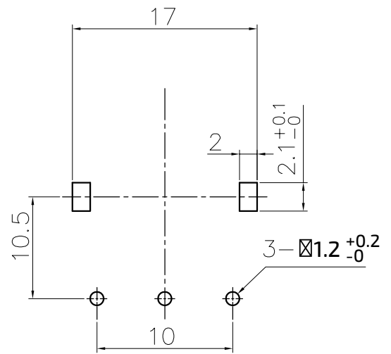
DETALHE MONTAGEM PCB
