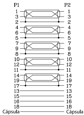
Distribuição dos pinos
